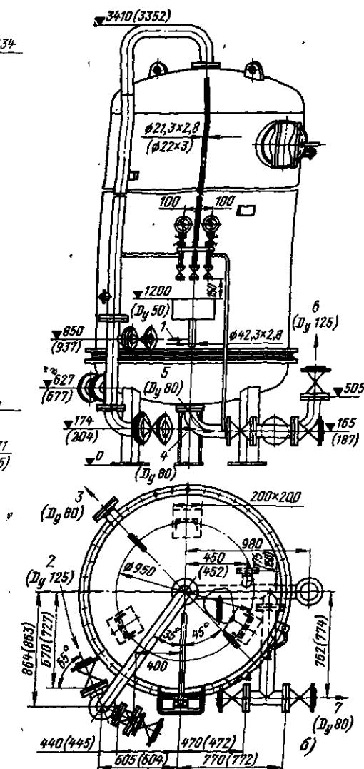
а — фильтр диаметром 1000 мм; б — фильтр диаметром 1400 мм; 1 — подвод регенерационного раствора; 2 — подвод обрабатываемой воды; 3 — штуцер для гидровыгрузки, установлен на отметке 770 и 925 мм; 4 — спуск промывочной воды; 5 — подвод промывочной воды; 6 — выход обработанной воды; 7 — спуск отмываемой воды.
