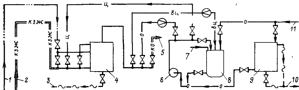
Рис. 2-17. Схема обезжелезивания конденсата в целлюлозных фильтрах намывного типа. 1 — сжатый воздух; 2 — зажелезенный конденсат; 3 — сброс целлюлозы в золоотвал; 4 — целлюлозный намывный фильтр; 5 — обезжелезенный конденсат; 6 — насос для намыва целлюлозы; 7 — загрузка целлюлозы; 8 — гидроразбиватель целлюлозы; 9 — бак осветленной воды; 10 — дренаж; 11 — осветленная вода.
