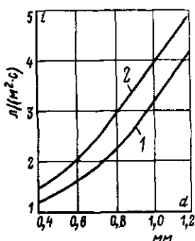
Рис. 5-4. График для определения необходимой интенсивности взрыхления катионита l в зависимости от диаметра зерен катионита d .
