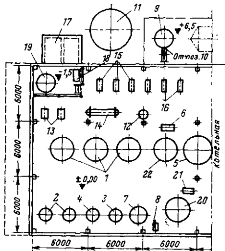
Рис. 9-6. Компоновка водоподготовительной установки по схеме рис. 9-5 с водород-катионитными фильтрами диаметром 2600 мм и натрий-катионитными фильтрами диаметром 1500 мм.
