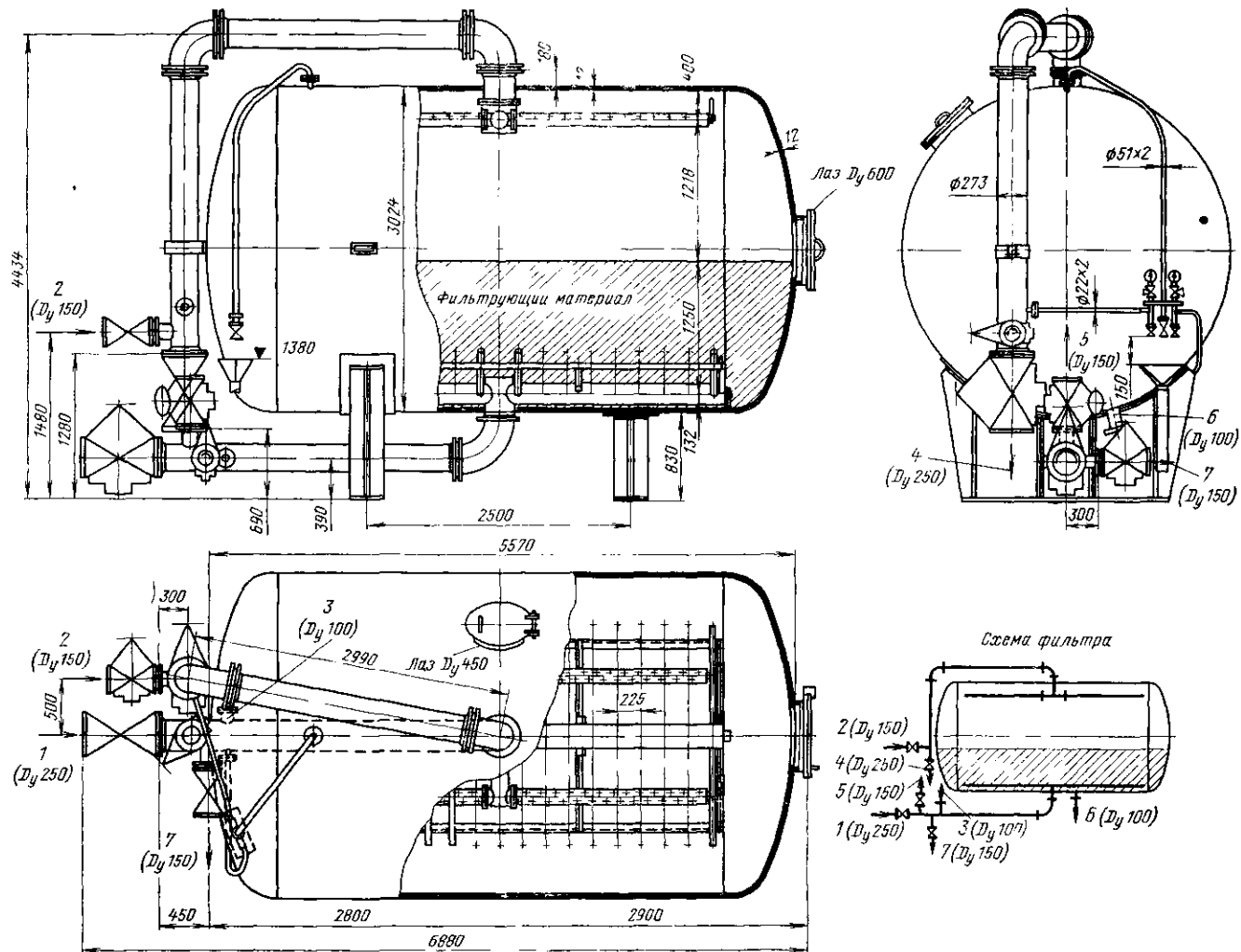
Рис. 7-7. Фильтр осветлительный горизонтальный диаметром 3000 мм, L = 5570 мм (ТКЗ).
