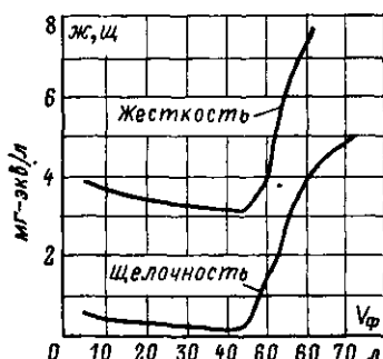
Рис. 2-6. График изменения жесткости и щелочности (Щ, Ж) в процессе водород-катионирования с «голодной» регенерацией фильтров в зависимости от объема фильтрата ( V_{\phi} ). Качественные показатели исходной воды:
