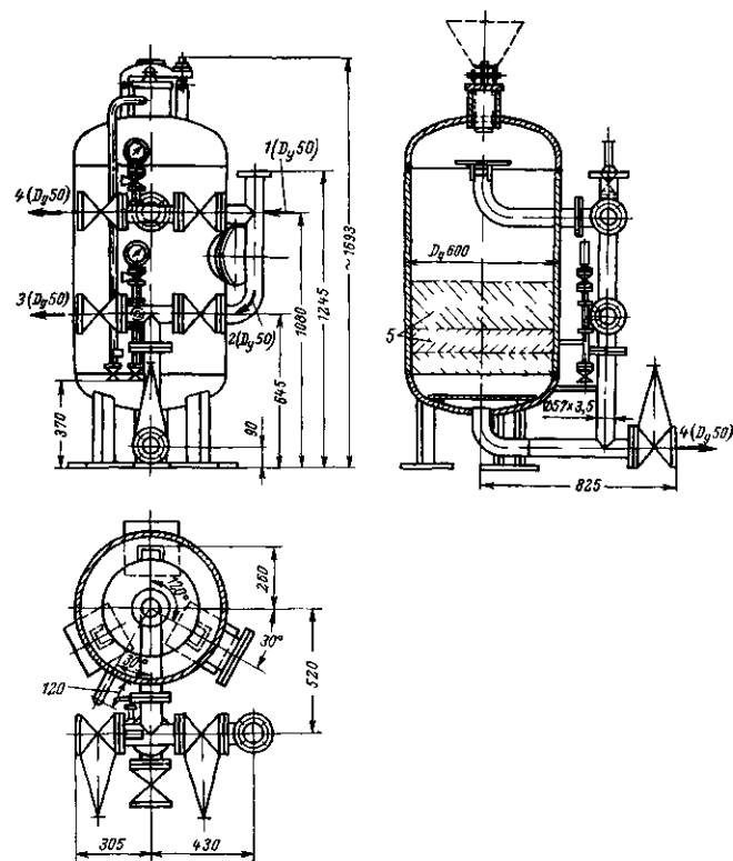
Рис. 7-57. Солеарастовитель реагентов D_y = 600 мм (СЗТМ).
