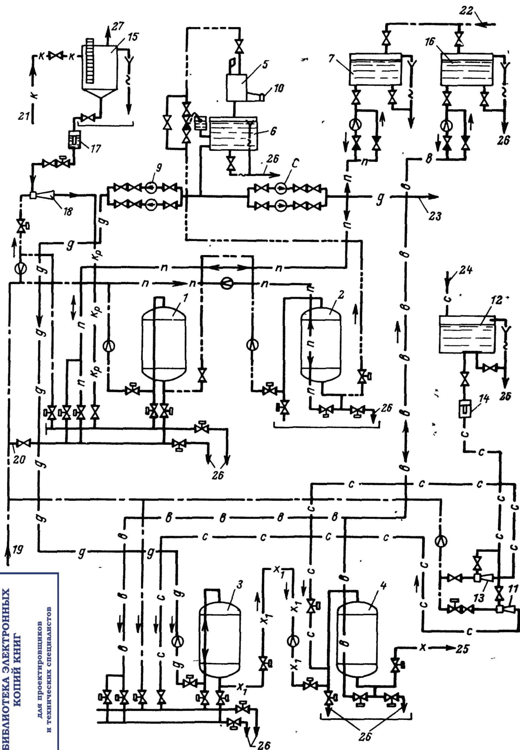
Рис. 10-5. Схема автоматизированной водоподготовительной установки.
