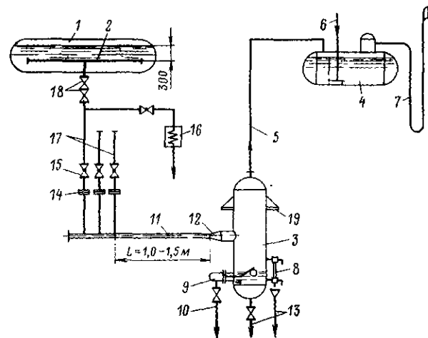
Рис. 14-3. Схема непрерывной продувки с установкой сепаратора D_y = 300 Бийского котельного завода.
