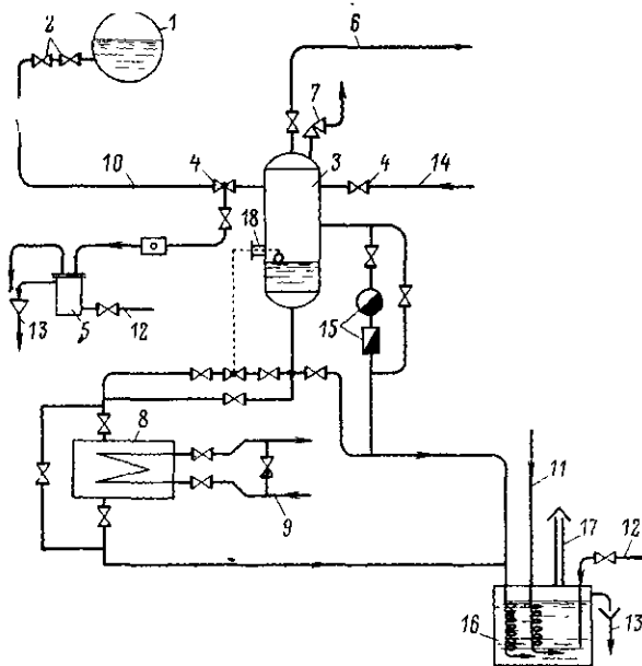
Рис. 14-2. Принципиальная схема непрерывной продувки котла с использованием тепла продувочной воды.
