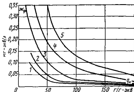
Рис. 5-5. Определение удельного расхода серной кислоты q_k в зависимости от требуемой жесткости фильтрата Ж_ф и общего солевого содержания исходной воды.
