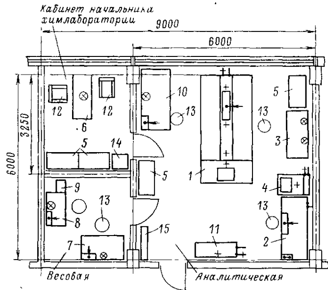
Рис. 12-2. Компонировка оборудования химической лаборатории типа I.
