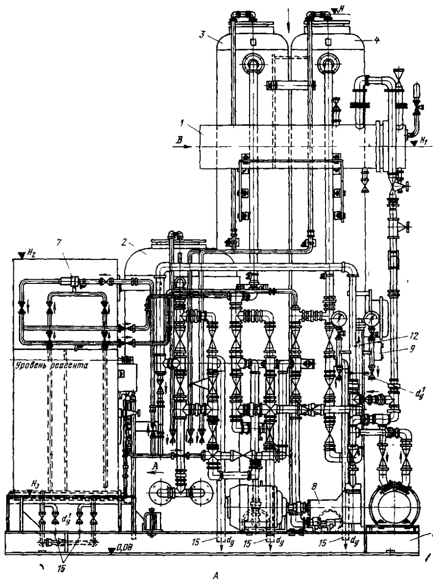
Рис. 7-47. Компонка блочных водоподготовительных установок производительности 5 и 10 м³/ч (СЗТМ), см. табл. 7-24.
