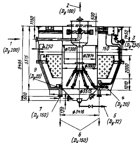
Рис. 8-4. Осветлитель для коагуляции воды типа ЦНИИ-3 (автор Е. Ф. Кургаев) производительностью 150 м³/ч.
