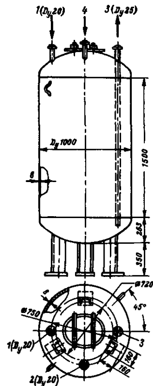
Рис. 7-31. Бак-вытеснитель крепкой серной кислоты емкостью 1,5 м 3 (БКЗ).
