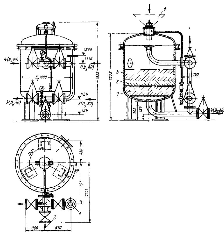
Рис. 7-58. Солеарастовитель реагентов D_y = 1000 мм (СЗТМ).
