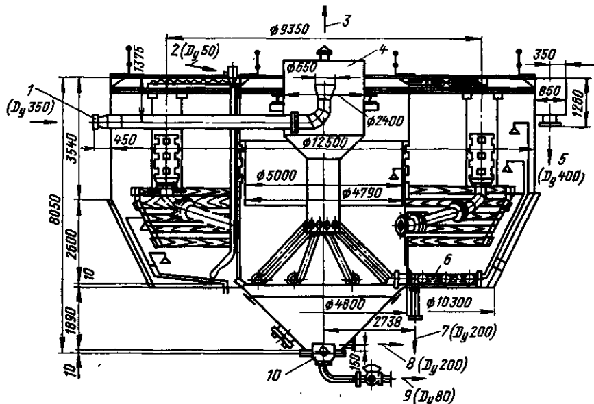
Рис. 8-6 Осветлитель для коагуляции воды типа ЦНИИ-3 (автор Е. Ф. Кургаев) производительностью 450 м 3 /ч.
