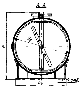
Рис. 7-59. Баки (опытные) для хранения серной кислоты и щелочи, V = 16, 32 и 40 \text{ м}^3 с подогревом (ТКЗ).
