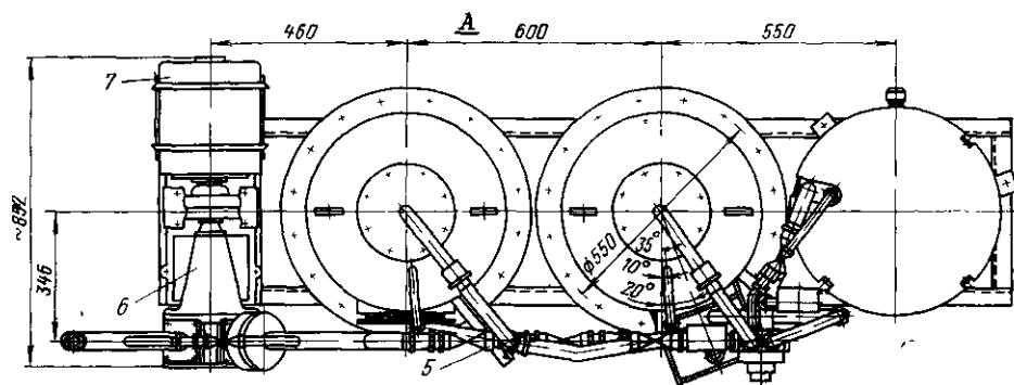
Рис. 7-48. Компонка оборудования блочной водоподготовительной установки с осветлительным фильтром производительностью 1,0 м³/ч (ММЗ).
