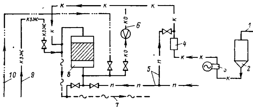
Рис. 2-18. Схема обезжелезивания конденсата на водород-катионитных фильтрах, загруженных сульфоуглем.
