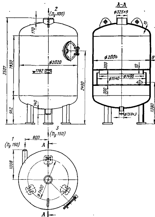
Рис. 7-44. Расширитель периодической продувки СП-7,5 (ТКЗ).
