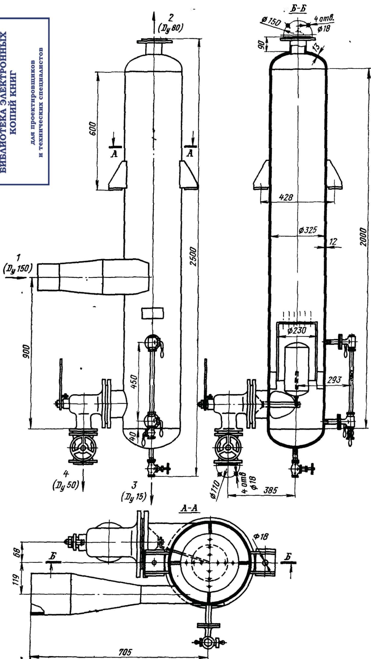
Рис. 7-40. Сепаратор непрерывной продувки D_y = 300 мм (со сферическим днищем), БикЗ. 1 — подвод продувочной воды; 2 — выход пара; 3 — спуск; 4 — выход отсепарированной воды.
