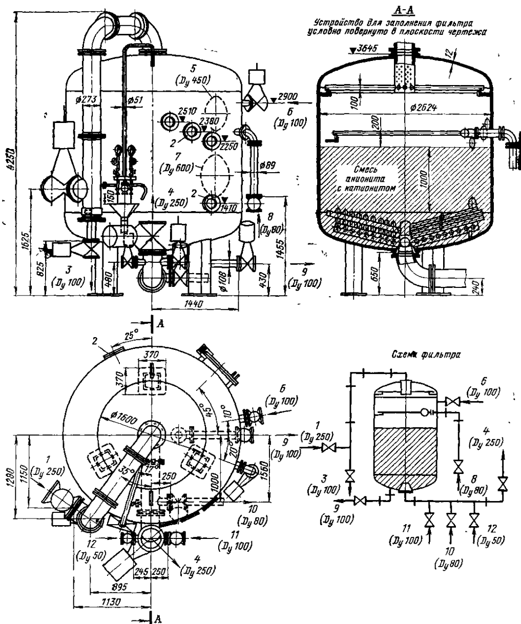
Рис. 7-22. Фильтр смешанного действия (ФСД) диаметром 2600 мм с выносной регенерацией (ТКЗ).
