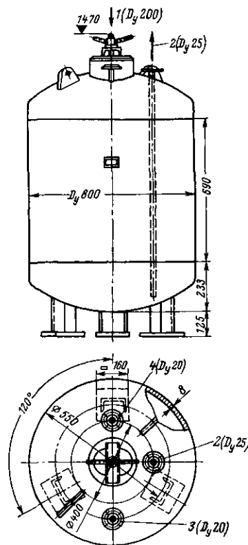
Рис. 7-30. Бак-вытеснитель крепкой серной кислоты емкостью 0,5 м 3 (БКЗ).
