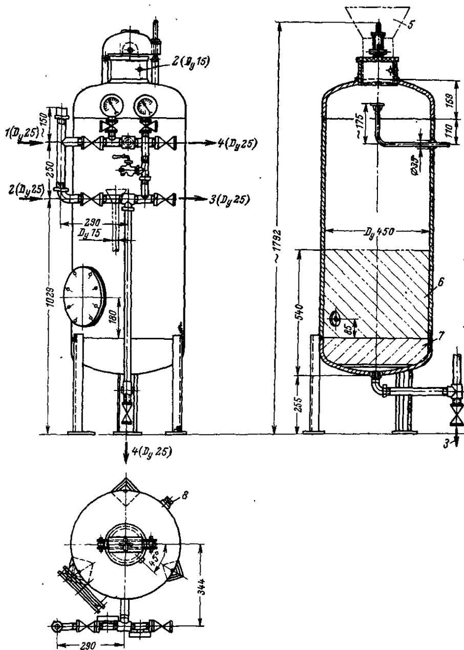
Рис. 7-56. Содерастворитель реагентов D_y \approx 450 мм (СЗТМ).
