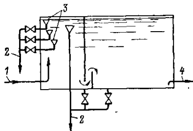
Рис. 2-13. Бак-отстойник конденсата.
