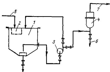
Рис. 6-4. Схема приготовления раствора коагулянта в гидравлической мешалке.
