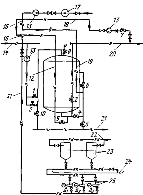
Рис. 5-8. Схема автоматизации противоточного водород-катионитного фильтра.
