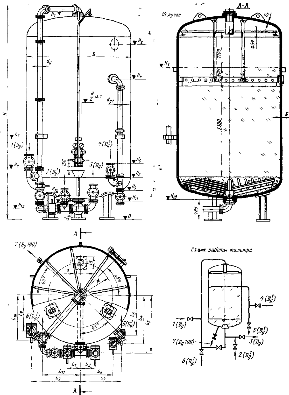
Рис. 7-19. Фильтры ионообменные противоточные водород-катионитные с „зажатым слоем“ диаметром от 2000 до 3400 мм (ТКЗ), см. табл. 7-13.
