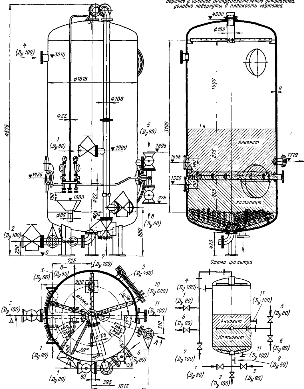
Рис. 7-24. Регенератор диаметром 1600 мм к ФСД-2,0 (ТКЗ);
