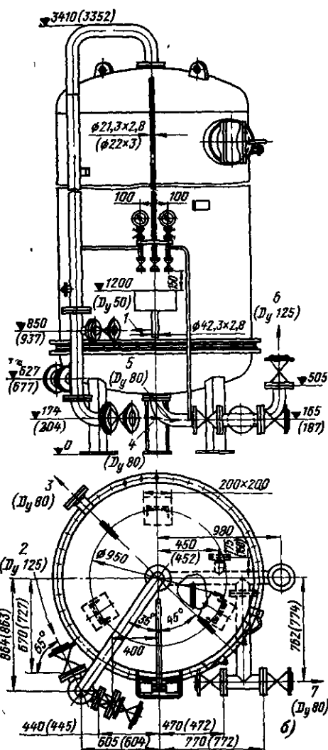
Рис. 7-16. Фильтры натрий- и водород-катионитные второй ступени (нижнее распределительное устройство — ложное дно выполнено из пресс-материала АГ-4с), БИКЗ.
