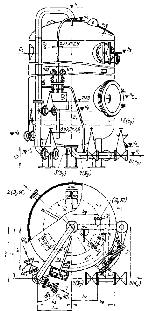
Рис. 7-11. Фильтры натрий-катионитные первой ступени диаметром 1000 и 1500 мм (БикЗ), см. табл. 7-6.
