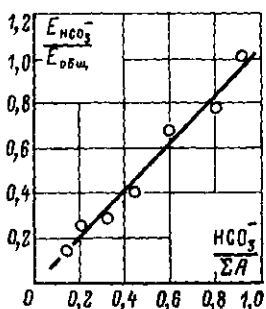
Рис. 2-4. Соотношение бикарбонатной и общей обменной емкости поглощения при различных соотношениях в исходной воде бикарбонат-ионов к сумме анионов сильных кислот.
