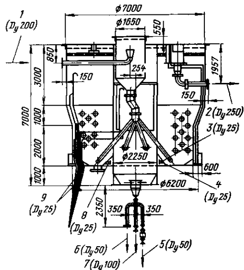
Рис. 8-3. Осветлитель для коагуляции воды производительностью 100 м³/ч.
