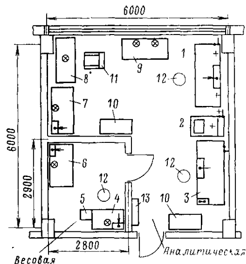
Рис. 12-3. Компонировка оборудования химической лаборатории типа II.
