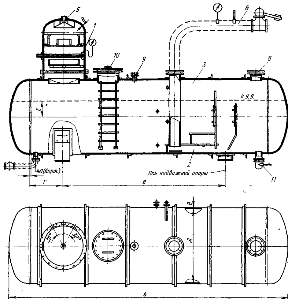
Рис. 13-5. Общий вид двухступенчатого деаэратора атмосферного давления (основные габаритные размеры — см. табл. 13-3).
