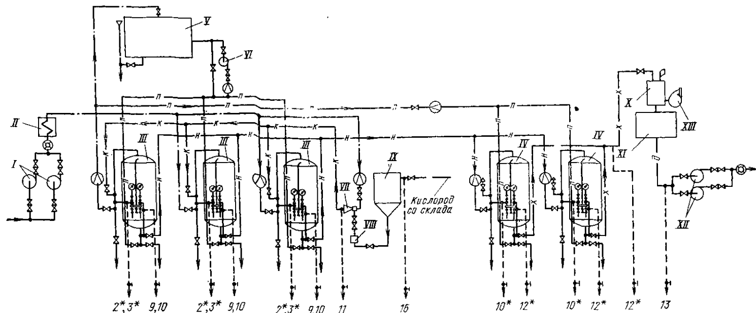
Рис. 12-1. Схема пробоотборных точек установки водород-катионирования с „голодной“ регенерацией фильтров.
