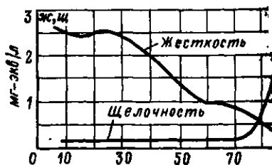
Рис. 2-7. График изменения жесткости и щелочности фильтрата (Щ, Ж) в процессе водород-катионирования с «голодной» регенерацией фильтров в зависимости от объема фильтрата ( V_{\phi} ). Качество исходной J_{\text{ж}} = 8 \text{ мг-экв/л} ; \text{Щ}_{\text{и.в.}} = 7,2 \text{ мг-экв/л} ; A = 2,6 .
