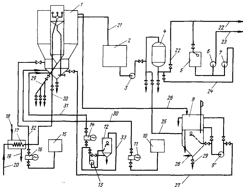
Рис. 10-2. Принципиальная схема установки предварительной обработки воды (пред-очистка).
