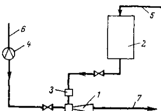
Рис. 6-10. Схема приготовления регенерационного раствора.
