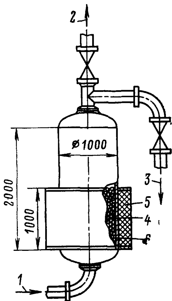
Рис. 2-19. Схема электромагнитного фильтра, заполненного стальными шариками.
