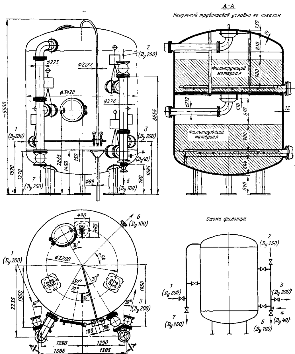
Рис. 7-4. Фильтр осветительной двухкамерный диаметром 3400 мм (ТКЗ).
