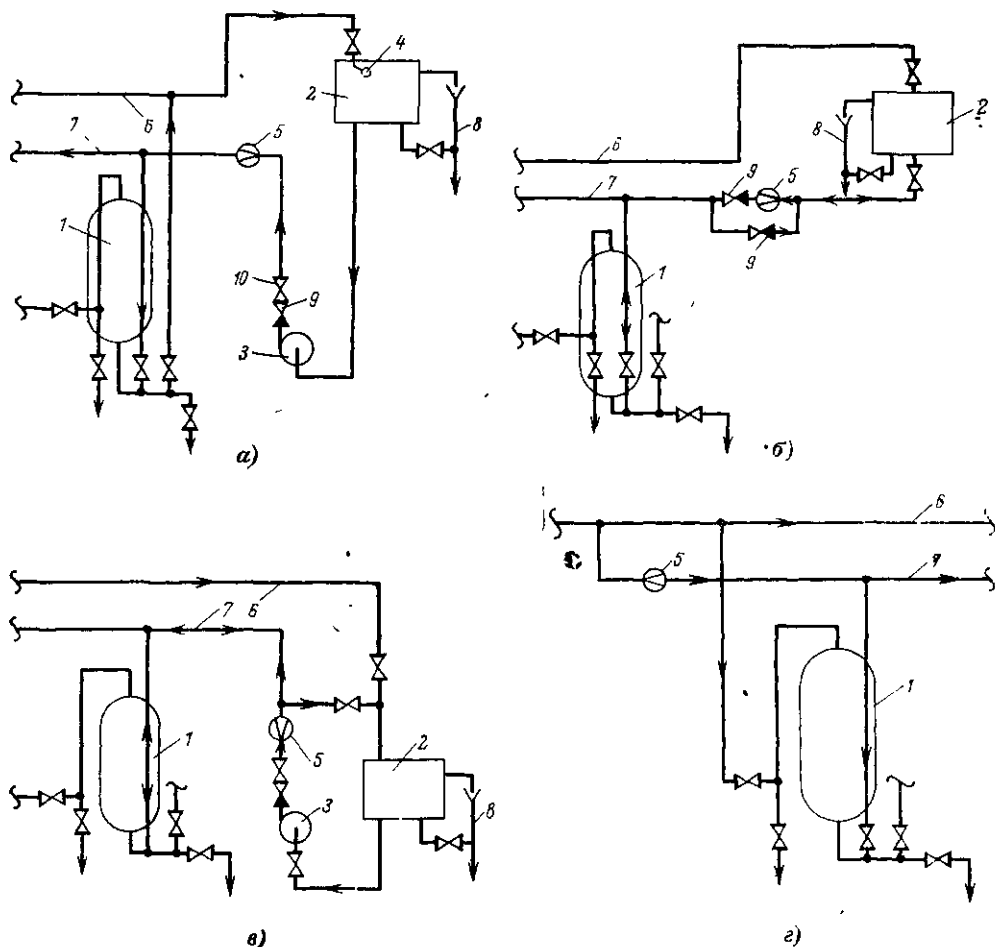
Рис. 6-9. Схема взрыхляющей промывки фильтров.
