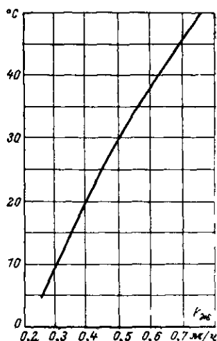
Рис. 5-10. График зависимости коэффициента десорбции k_{ж} от температуры для декарбонизаторов, загруженных кольцами Рашига 25 \times 25 \times 3 мм, при плотности орошения насадки 60 м^3/(м^2 \cdot ч) .
