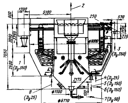
Рис. 8-5. Осветлитель для коагуляции воды типа ЦНИИ-3 (автор Е. Ф. Кургаев) производительностью 230 м³/ч.
