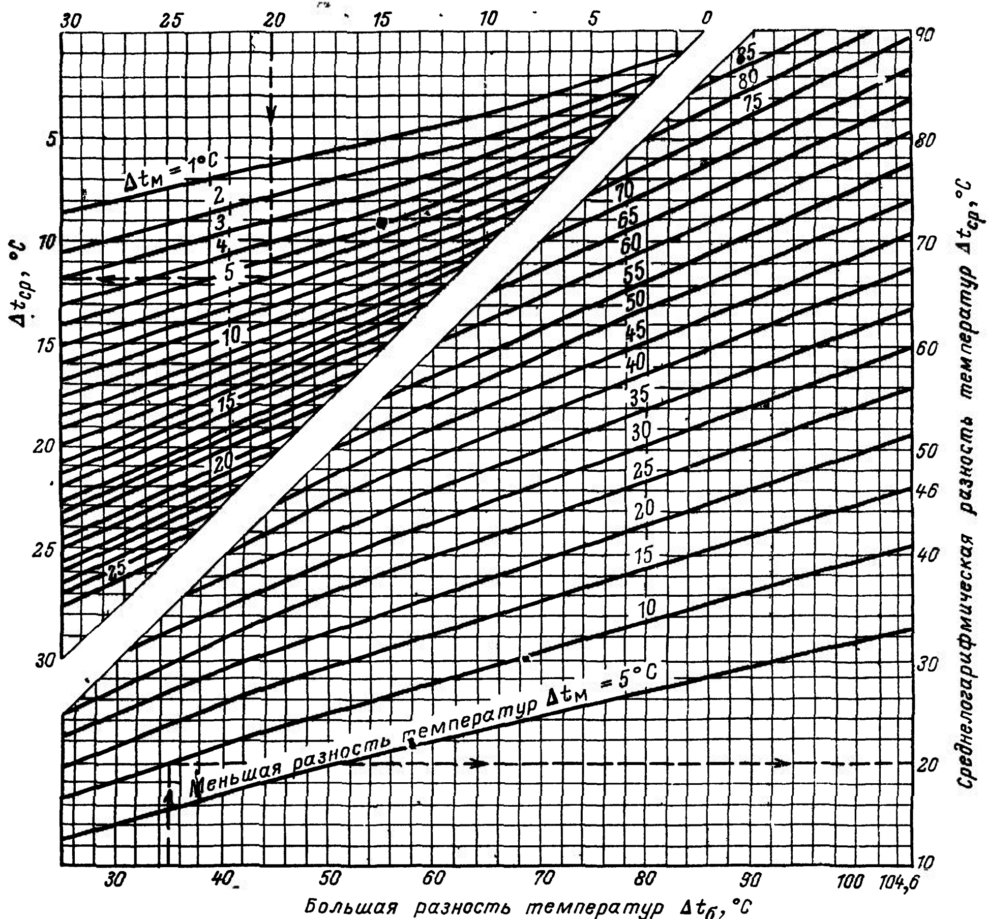
Рис. 14-4. График определения среднеарифметической разности температур.
