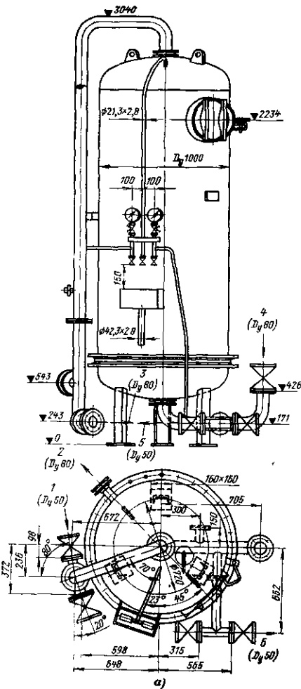
Рис. 7-2. Фильтры осветительные (нижнее распределительное — ложное дно из пресс-материала АГ-4С), БИКС.
