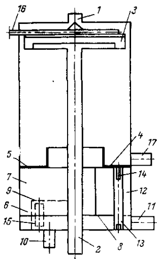
Рис. 13-6. Принципиальная схема вакуумного барботажного деаэратора.
