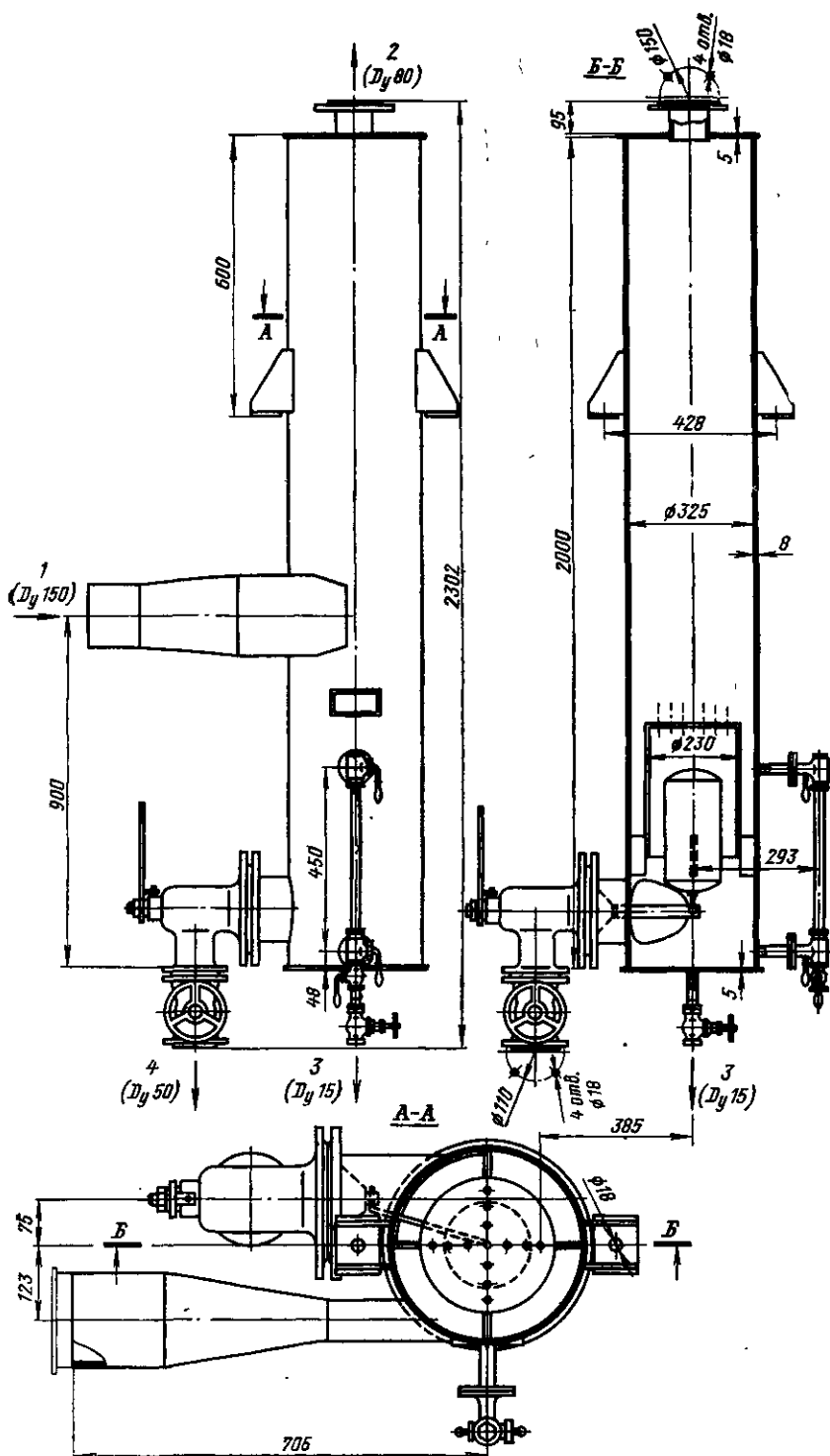
Рис. 7-39. Сепаратор непрерывной продувки D_y = 300 мм (с плоским дном), БЖЗ. 1 — подвод продувочной воды; 2 — выход пара; 3 — спуск; 4 — выход отсепарированной воды.
