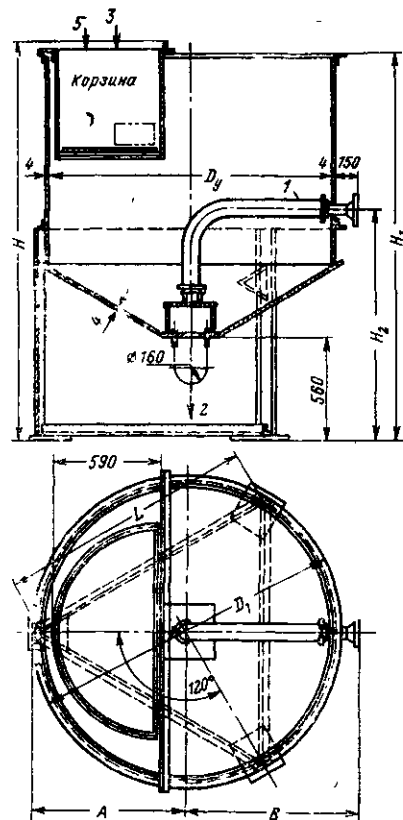
Рис. 7-29. Мешалки гидравлические для кислотных реагентов объемом 1 и 2 м 3 (ТКЗ), см. табл. 7-17а.
