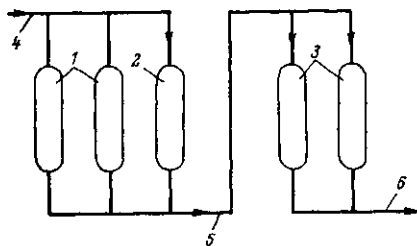
Рис. 9-7. Водоподготовительная установка для паровой котельной по схеме двухступенчатого натрий-катионирования с хлорированием.
