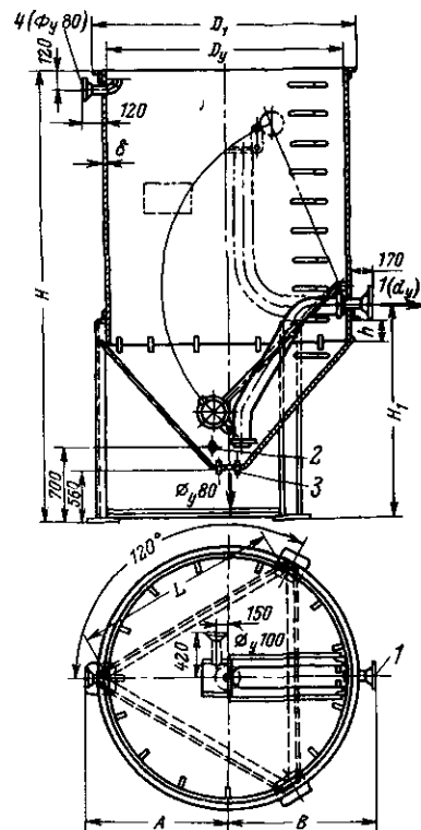
Рис. 7-28. Мешалки циркуляционные для известкового молока (ТКЗ), см. табл. 7-17.
