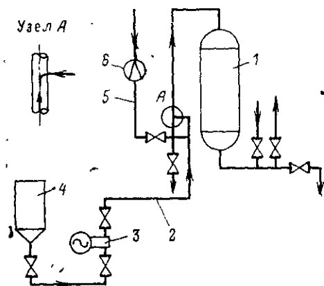
Рис. 6-11. Схема регенерации фильтра насосом-дозатором типа НД.
