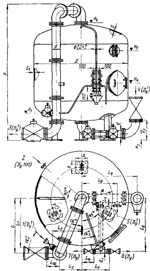
Рис. 7-3. Фильтры осветительные диаметром от 2000 до 3400 мм (ТКЗ), см. табл. 7-3.
