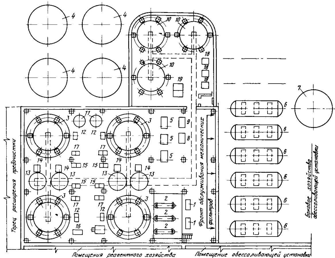
Рис. 9-9 Компоновка установки предварительной очистки (предочистки) поверхностной воды.
