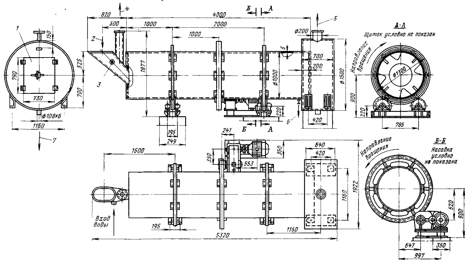
Рис. 7-54. Аппарат для гашения извести диаметром 1000 мм, производительностью 25 т/сут \text{CaO} .
