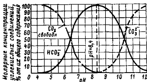
Рис. 10-4. График соотношений \text{CO}_2 , \text{HCO}_3^- и \text{CO}_3^{2-} в зависимости от pH воды.
