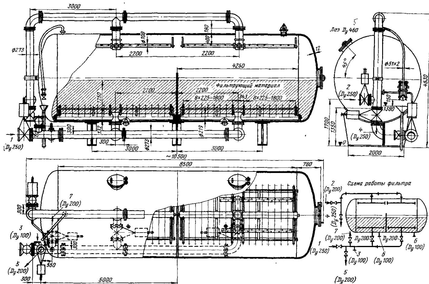
Рис. 7-б. Фильтр осветительный горизонтальный диаметром 3000 мм L = 10500 мм (ТКЗ):
