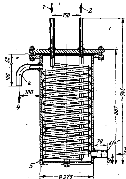
Рис. 7-45. Охладитель отбора проб пара и воды ЗН-249-67 (СЗТМ).
