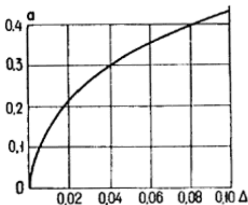
Черт.24. Номограмма зависимости между неравномерностью распределения воздуха \Delta и характеристикой трубопровода \alpha
