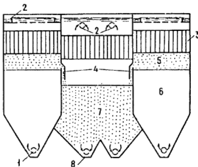
Черт.15. Осветлитель, оборудованный тонкослойными блоками
