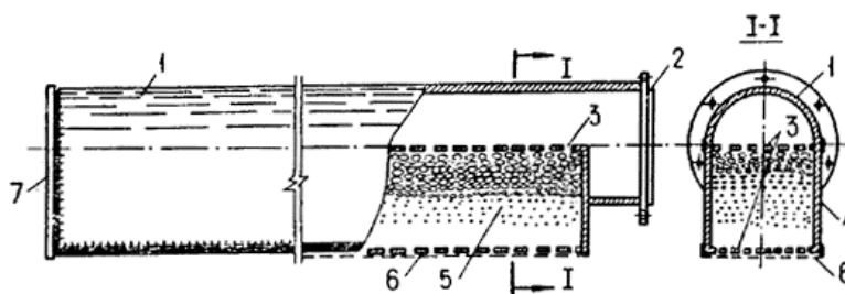
Черт.32. Конструкция среднего дренажа ФПЗ-4 (ФПЗ-4н)
