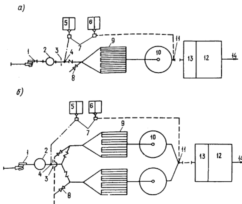
Черт.42. Принципиальная схема работы установок типа "Струя"
