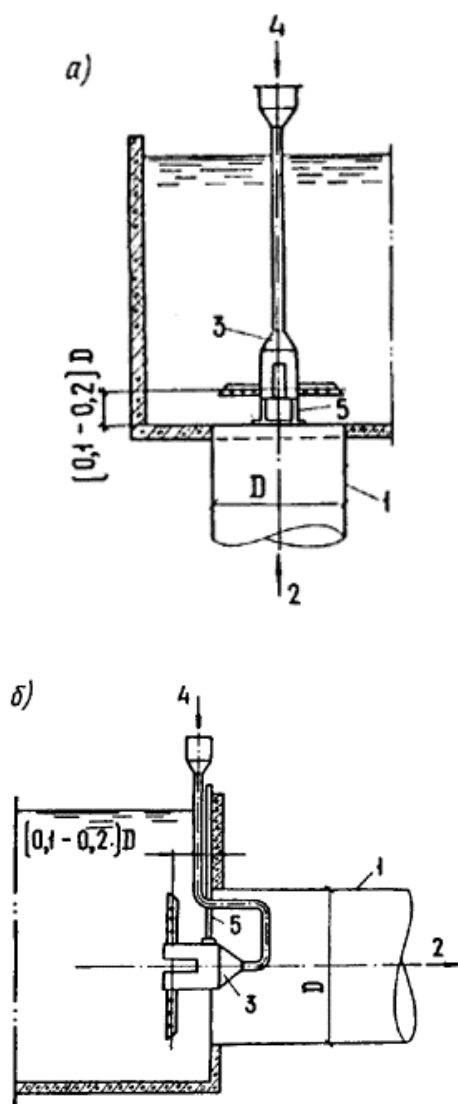
Черт.4. Схемы установки камерно-лучевых распределителей (тип II)
