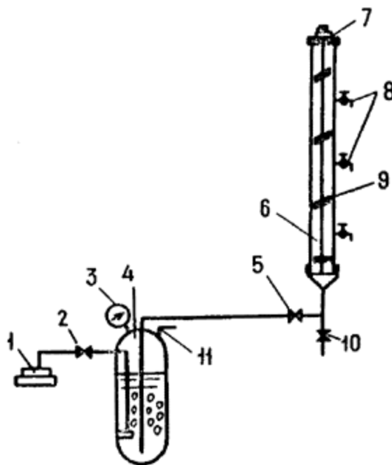
Черт.19. Установка для проведения технологического анализа воды
