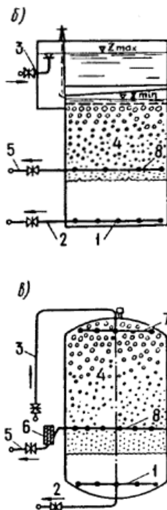
Черт.30. Фильтры с плавающей пенополистирольной загрузкой
