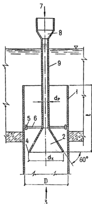
Черт.5. Диффузорный распределитель (тип III)
