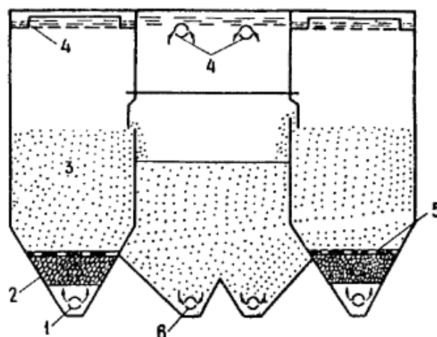
Черт.12. Осветлитель с контактной камерой хлопьеобразования
