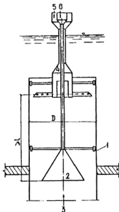
Черт.6. Схема совмещения диффузорного и камерно-лучевого распределителей
