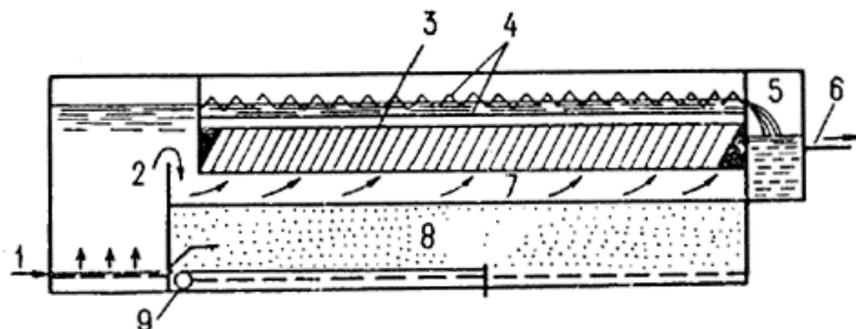
Черт.14. Горизонтальный отстойник, оборудованный тонкослойными блоками
