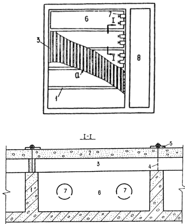
Черт.29. Дренаж из монолитного полимербетона
