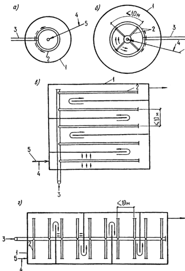
Черт.8. Трубчатые аэраторы
